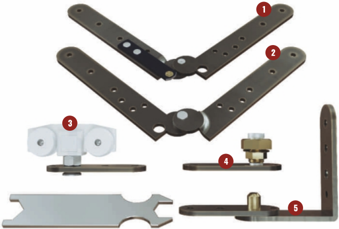
Комплект механизмов для дверей типа «Дверь-книжка»
