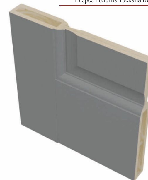
Разрез полотна Тоскана Neo
